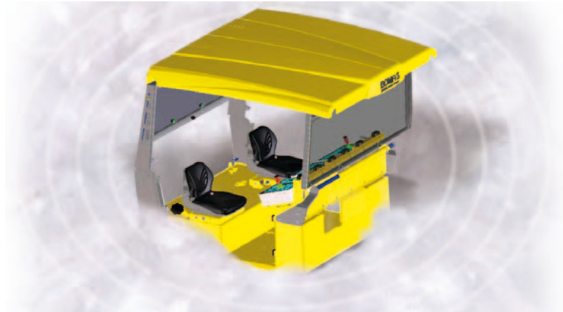
Виброизолированная платформа оператора.
